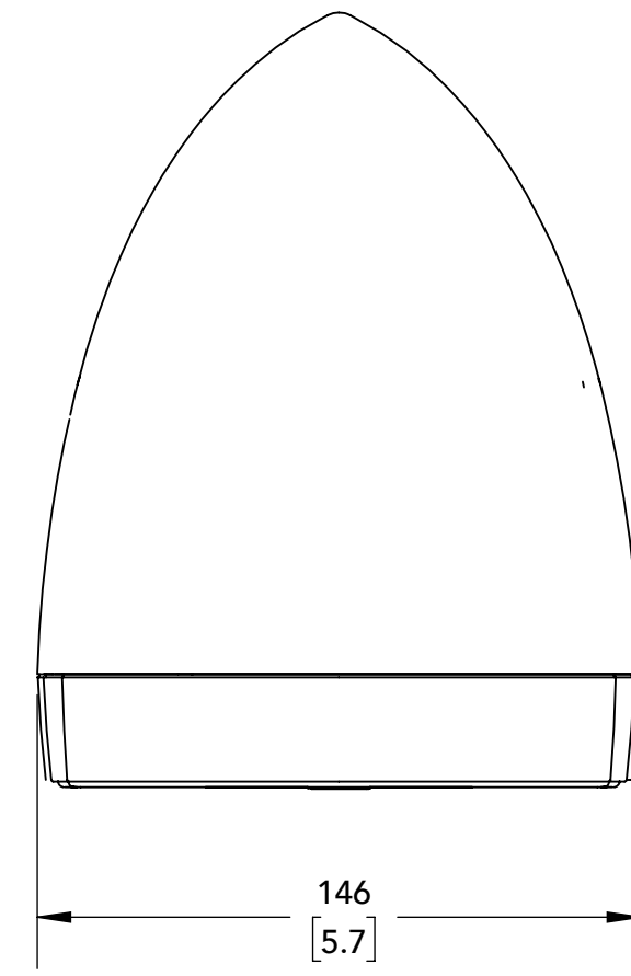
TOP
